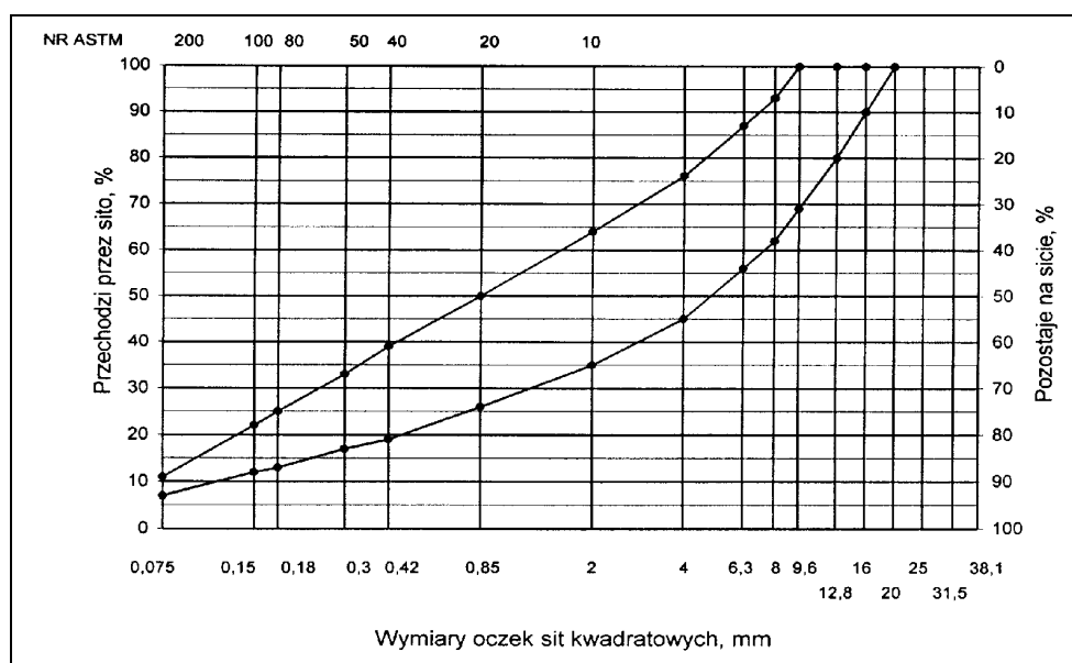
Rys. 2. Krzywe graniczne uziarnienia mieszanki mineralnej BA od 0 do 16mm, od 0 do 12,8 mm do warstwy ścieralnej obciążonej ruchem KR 1-2
