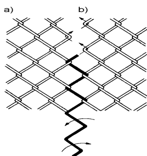
Rys. 2. Łączenie dwóch sąsiednich odcinków siatki za pomocą spirali wplecionej z siatki i wprowadzonej w oczka siatki ruchem śrubowym (wg [6])
