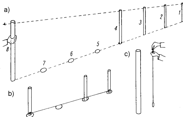
Rys. 4. Przykład ustawiania słupków ogrodzenia (wg [6])
