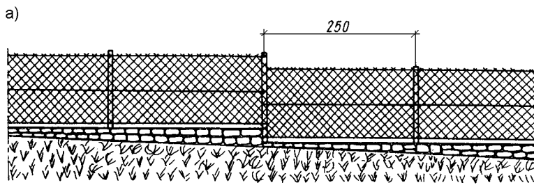
Rys. 6. Przykład ustawienia ogrodzenia siatkowego na terenie pochyłym (wg [6]) a) Ogrodzenie ze stopniami wysokości 25÷30 cm (przy spadku terenu od 1:16 do 1:30) b) Ogrodzenie równoległe do terenu
