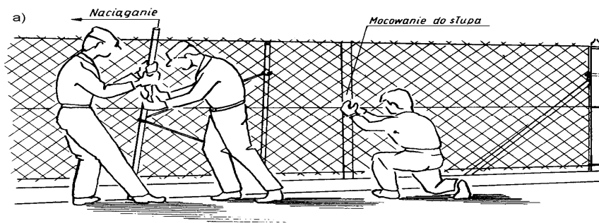
Rys. 8. Przykład napinania siatki przy ustawianiu ogrodzenia (wg [6])
