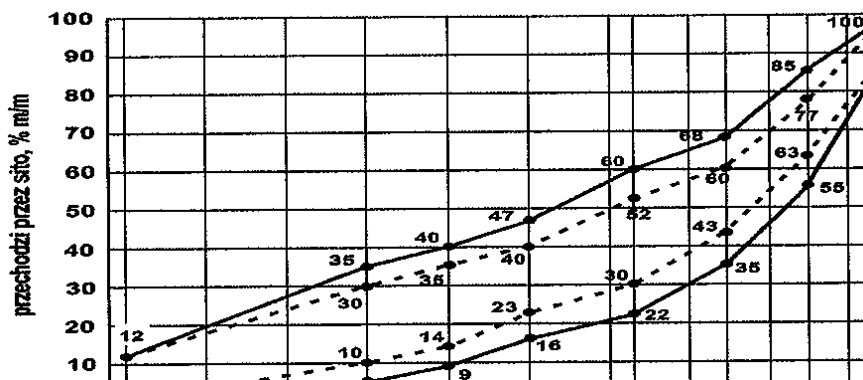
Rys. 1. Krzywe graniczne uziarnienia mieszanki kruszywa niezwiązanego, 0/45 mm
