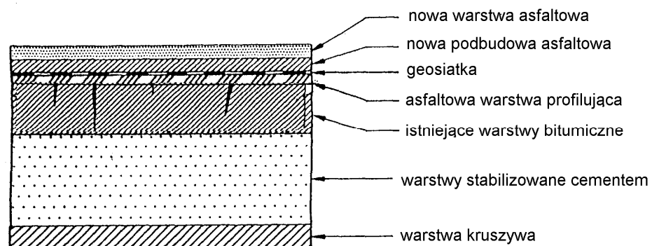
Rys. 7. Wzmocnienie nawierzchni asfaltowej położonej na istniejącej nawierzchni z betonu cementowego
