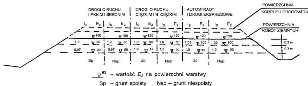
Rysunek 4 – Wartości wymagane w podłożu wykopów: wskaźnika zagęszczenia I_s i wrotnego modułu odkształcenia E_2 , megapaskali
