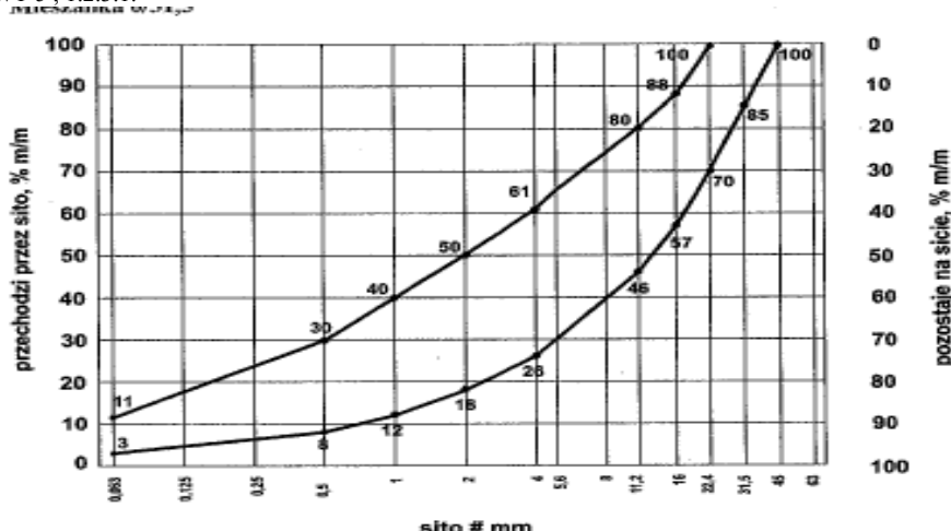
Rys.1.1. Uziarnienie mieszanki CBGM 0/31,5
