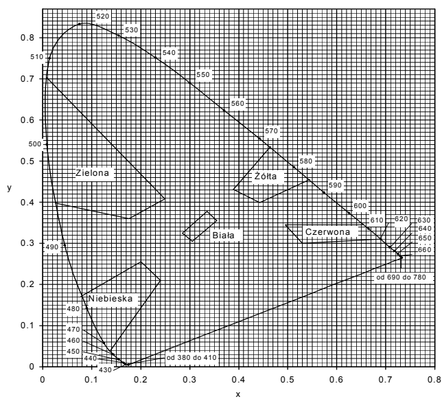
Rys.2. Współrzędne chromaticzności x,y dla barwy żółtej oznakowania
