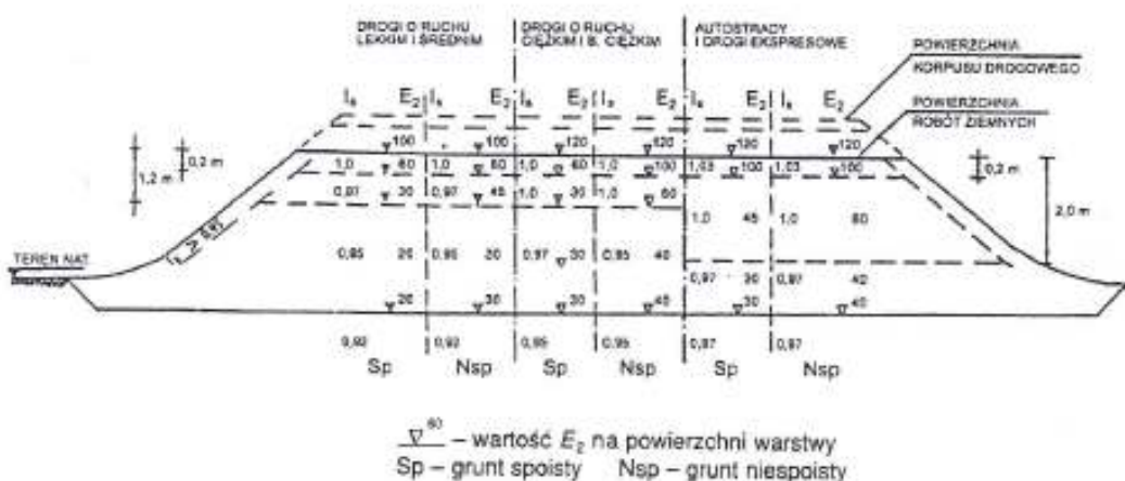
Rysunek 3 – Wartości wymagane w nasypach: Wskaźnika zagęszczenia I_2 i wtórnego modułu odkształcenia E_2 , megapaskall
